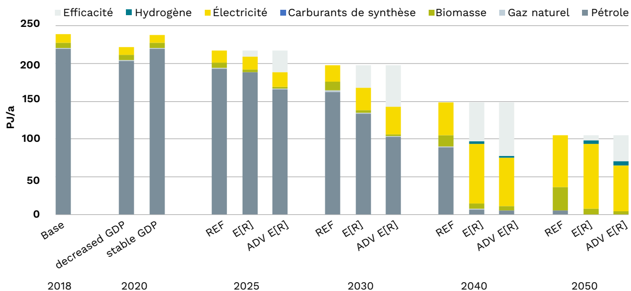
Illustration 5 : Evolution des sources d'énergie utilisées dans les transports. Efficacité = différence par rapport au scénario de référence.
