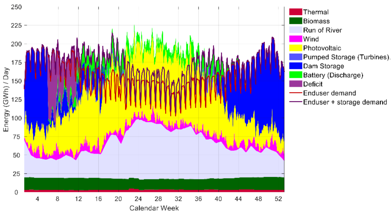
Illustration 9 : Modélisation de l'approvisionnement électrique autochtone de la Suisse en 2030 pour le scénario ADV. (Source : modèle énergétique SCS, résolution précise par jour, calculs Greenpeace)
