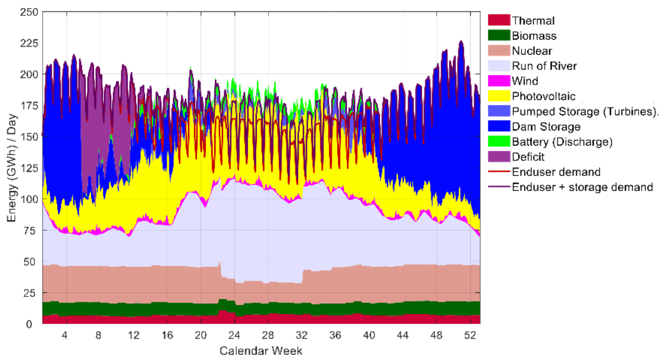
Illustration 8 : Modélisation de l'approvisionnement électrique de la Suisse en 2025 pour le scénario ADV. (Source : modèle énergétique SCS, résolution précise par jour, calculs Greenpeace)
