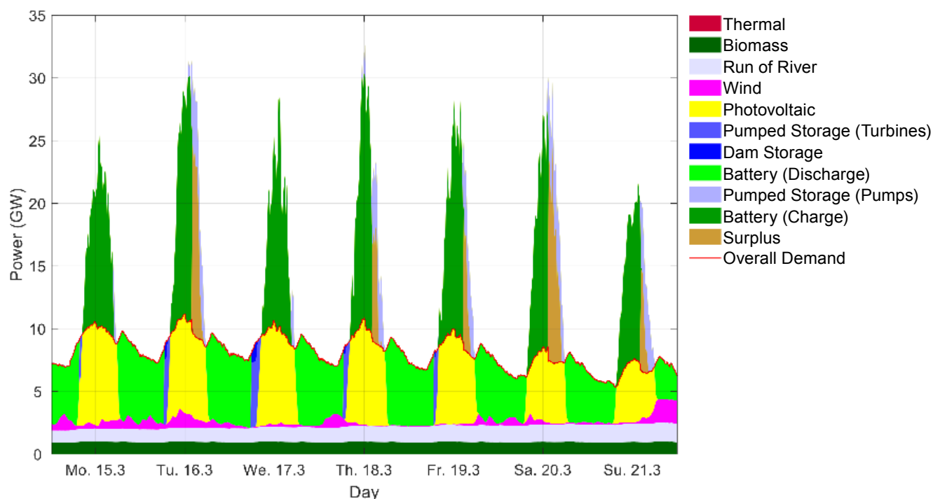
Illustration 12 : Répartition au quart d'heure de la production et de la consommation pour le scénario ADV pendant une semaine de printemps en 2050. (Source : modèle énergétique SCS, calculs Greenpeace)
