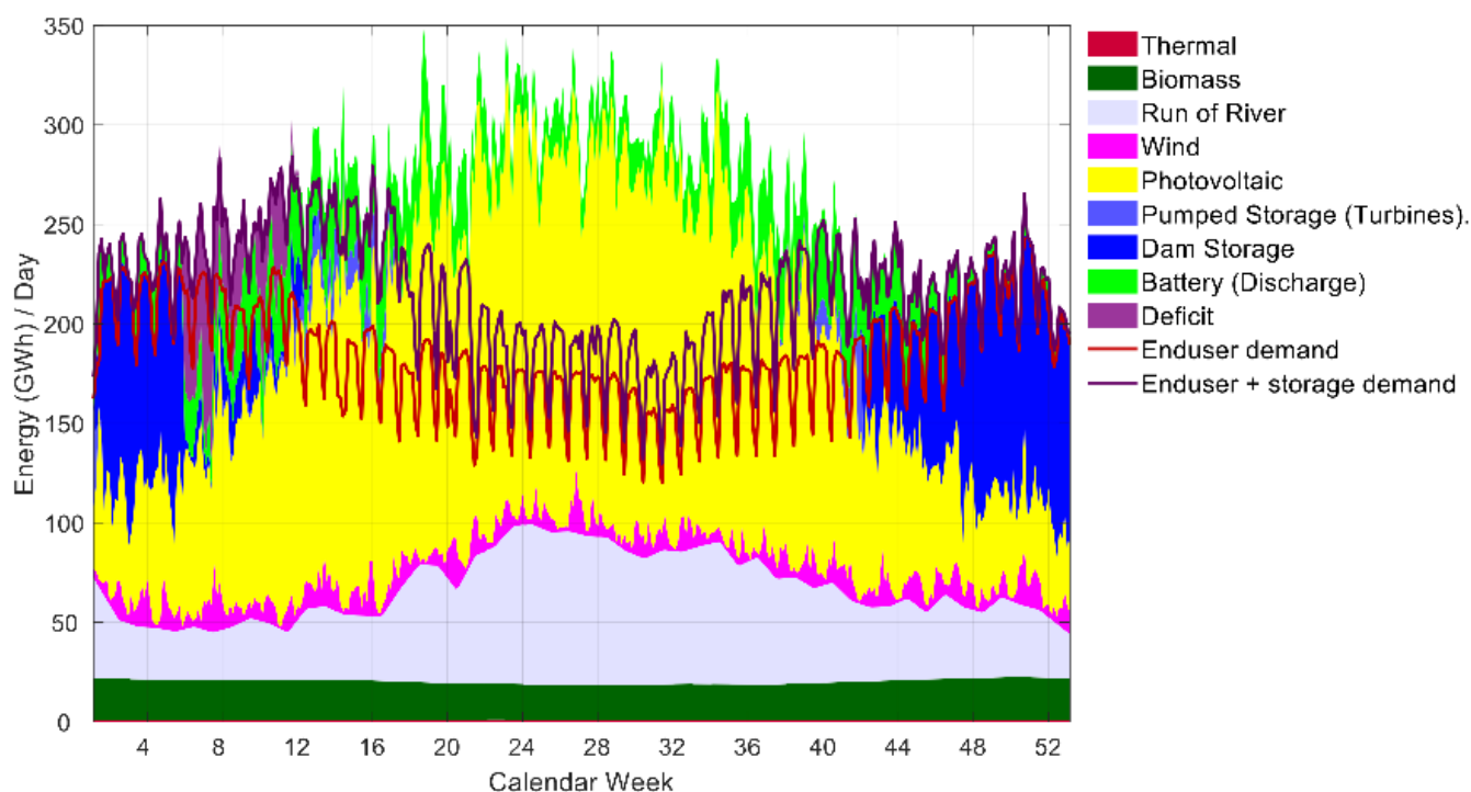
Illustration 10 : Modélisation de l’approvisionnement électrique de la Suisse en 2040 pour le scénario ADV. (Source : modèle énergétique SCS, résolution précise par jour, calculs Greenpeace)
