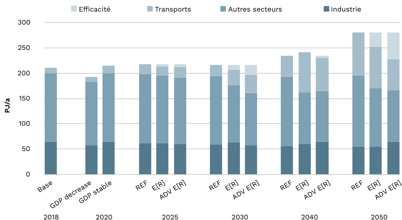
Illustration 6 : Évolution de la demande en électricité en fonction des secteurs, sans les pertes, avec autoconsommation pour le chargement de solutions de stockage et la production d'hydrogène. Efficacité = différence par rapport au scénario de référence.
